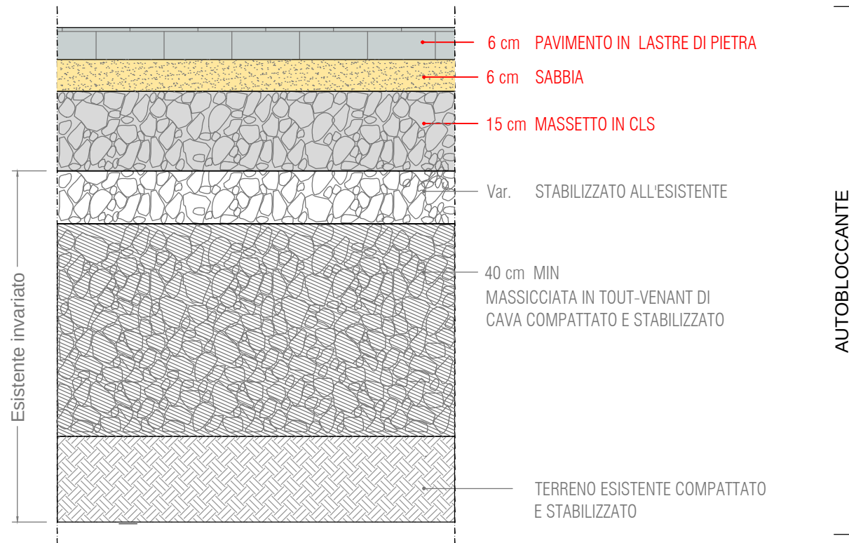
S5 - STRATIGRAFIA MARCIAPIEDE IN AUTOBLOCCANTE
