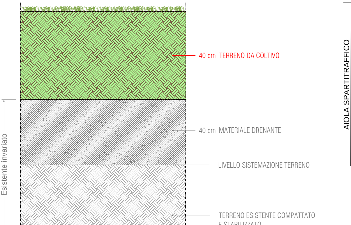
S7 - STRATIGRAFIA AIOLA SPARTITRAFFICO
