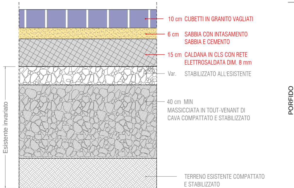
S6 - STRATIGRAFIA FASCIA SORMONTABILE IN PORFIDOE
