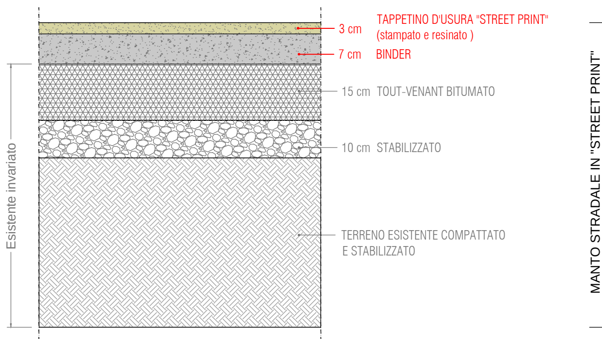
S2 - STRATIGRAFIA MANTO STRADALE STREET PRINT
