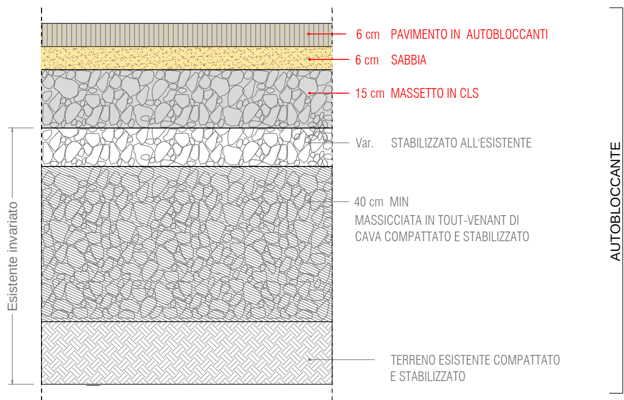
S4 - STRATIGRAFIA MARCIAPIEDE IN AUTOBLOCCANTE
