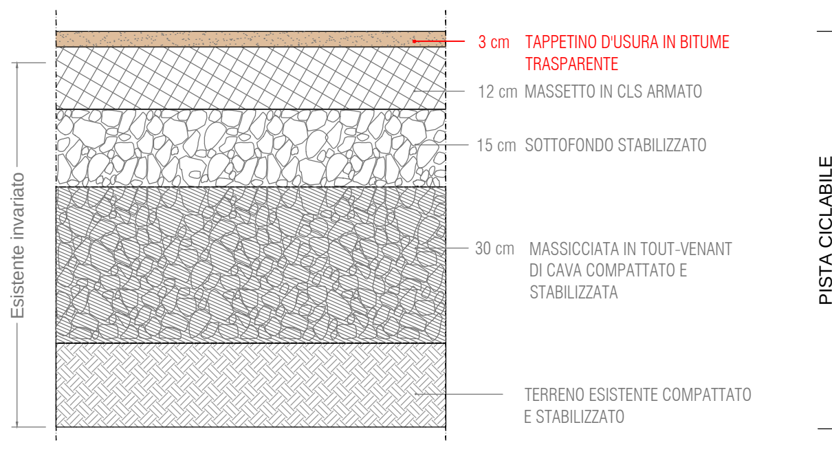
S3 - STRATIGRAFIA ASFALTO COLORATO /PISTA CICLABILE
