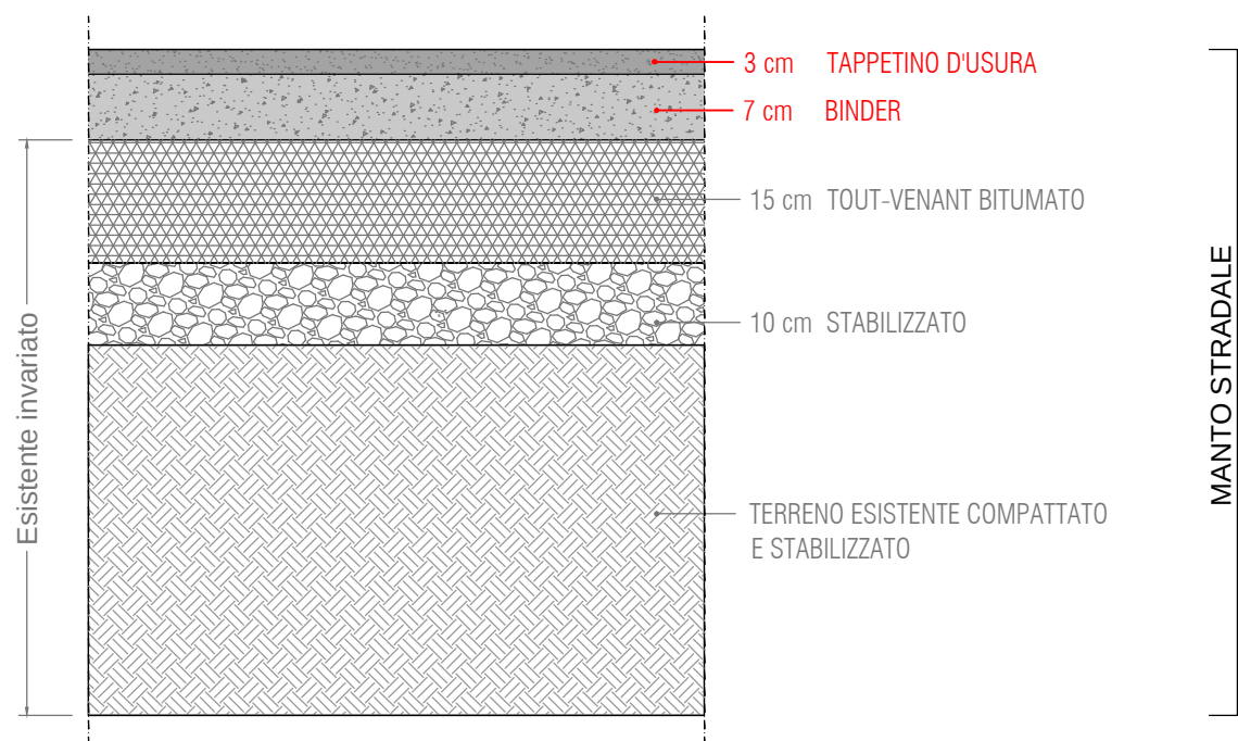
S1 - STRATIGRAFIA MANTO STRADALE
