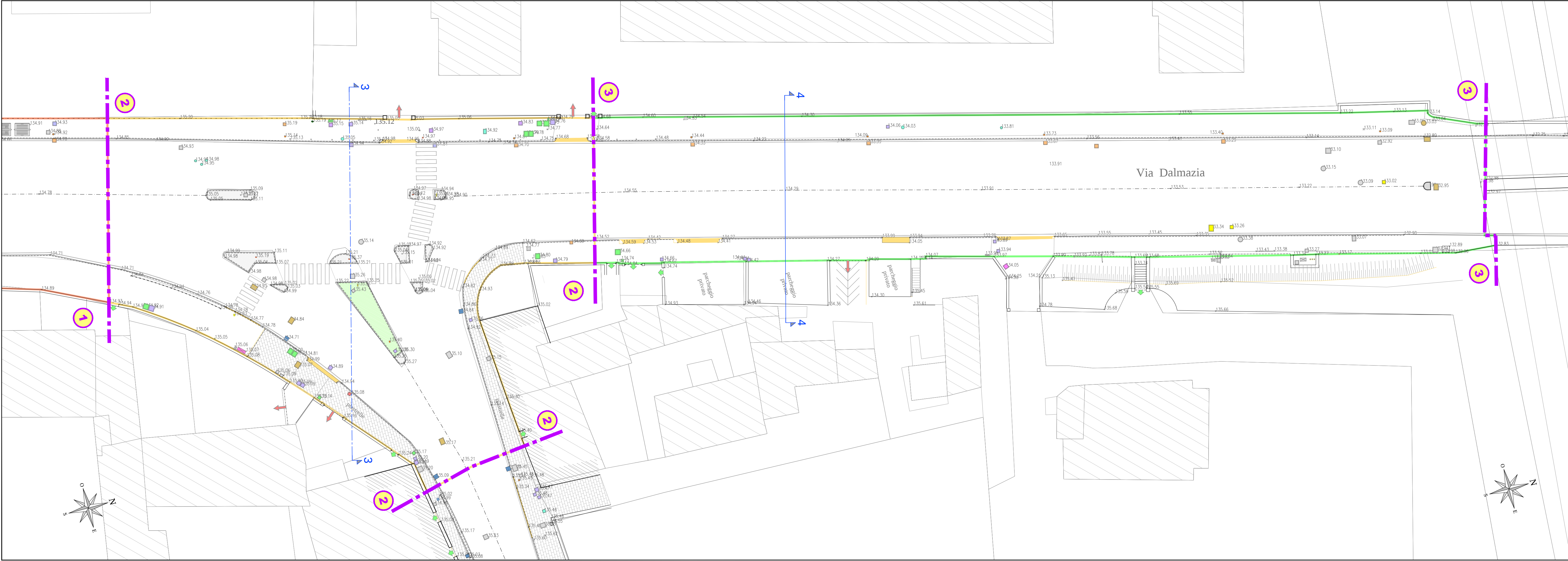
STATO DI FATTO - VIA San Giovanni BOSCO (Piazzale Papa Giovanni XXIII) - Intervento 4 (tavola 3 di 3)
