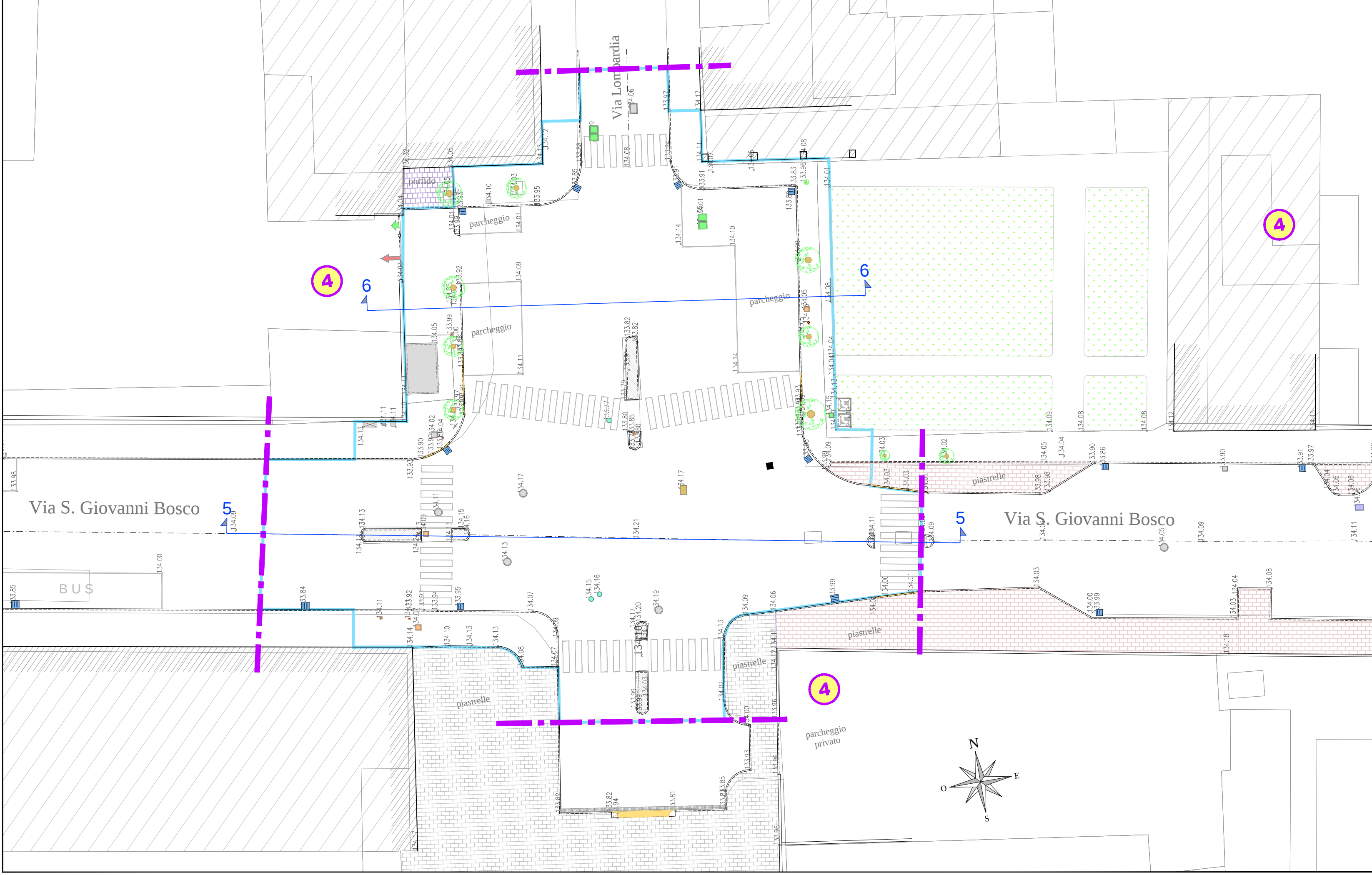
STATO DI FATTO - VIA San Giovanni BOSCO (Piazzale Papa Giovanni XXIII) - Intervento 4 (tavola 3 di 3)
