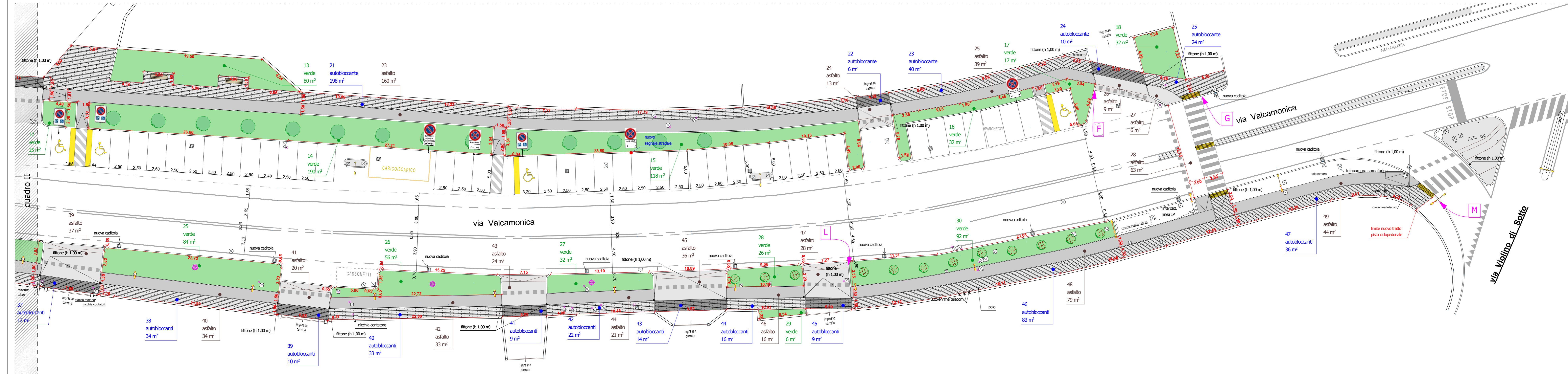
PLANIMETRIA DI PROGETTO - QUADRO III scala 1:200
