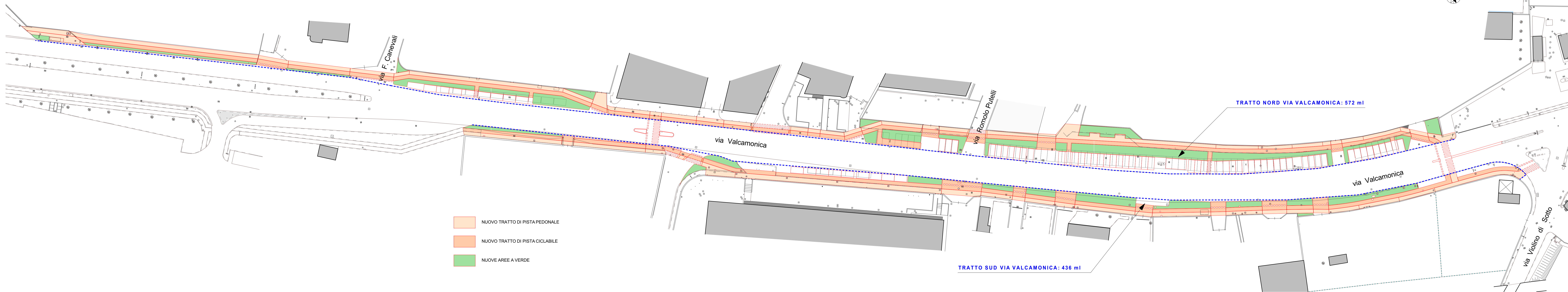
PLANIMETRIA GENERALE DELLO STATO DI FATTO scala 1:500
