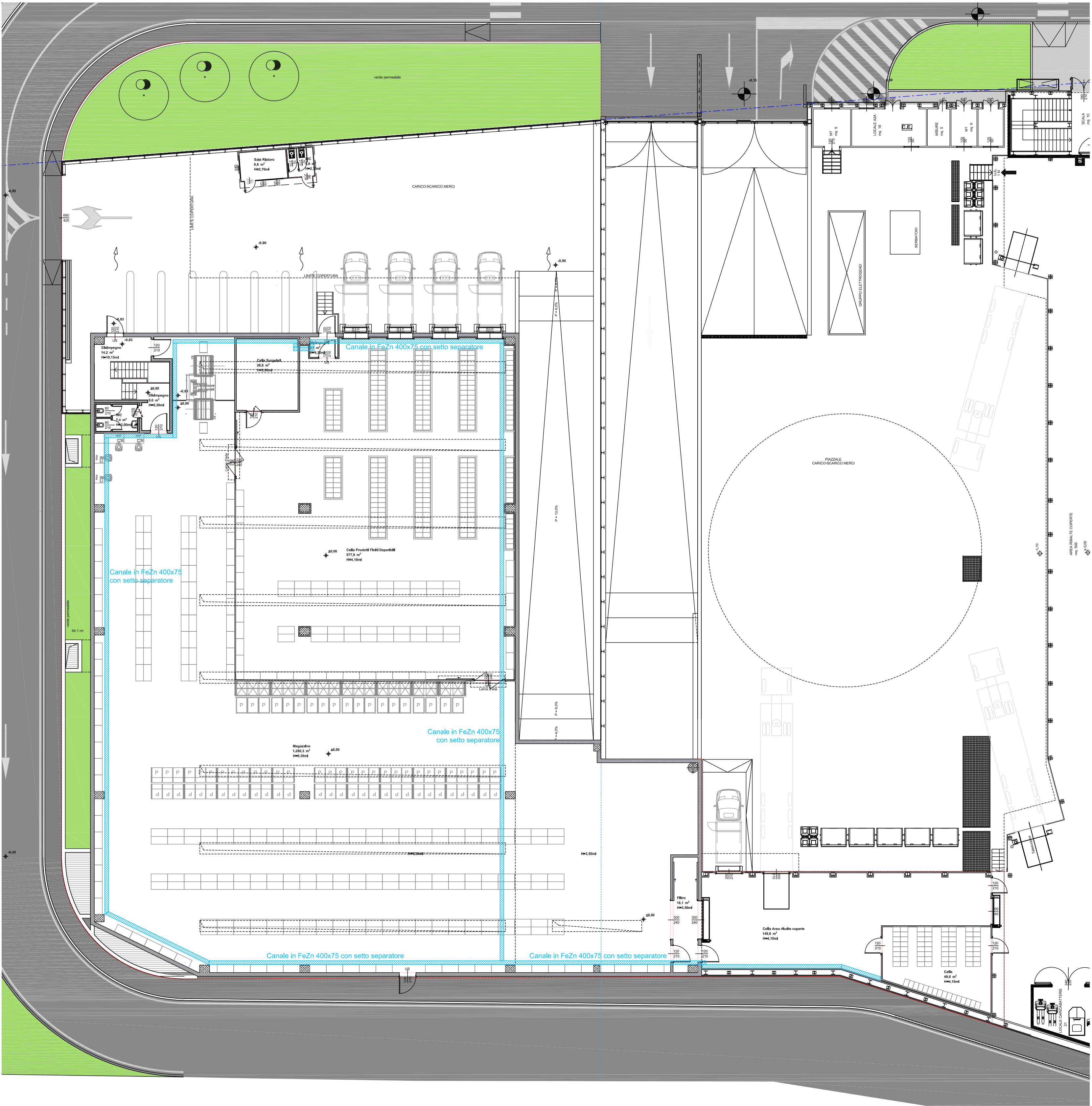
PIANO TERRA - Scala 1:200
