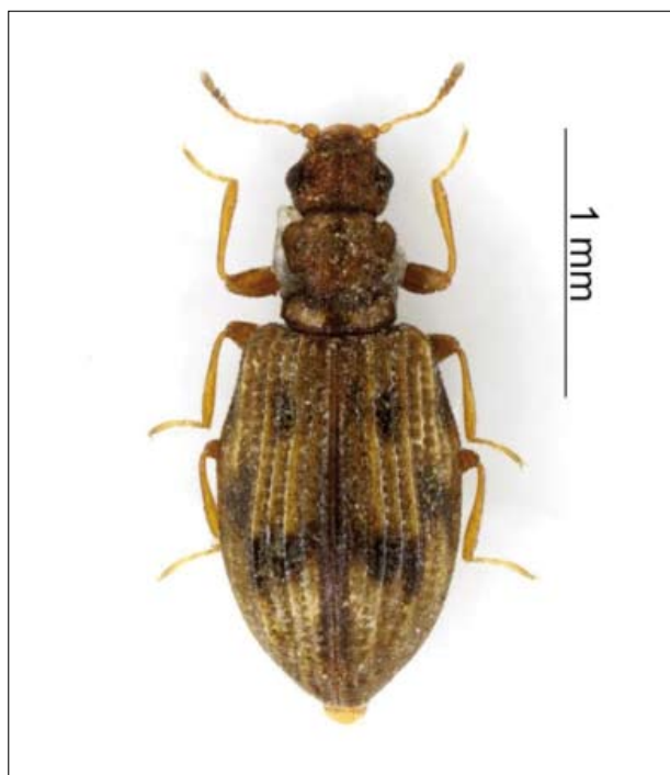
Fig. 1. Cartodere (Aridius) bifasciata , habitus (Emilia Romagna (BO), Mordano, loc. Bubano).
