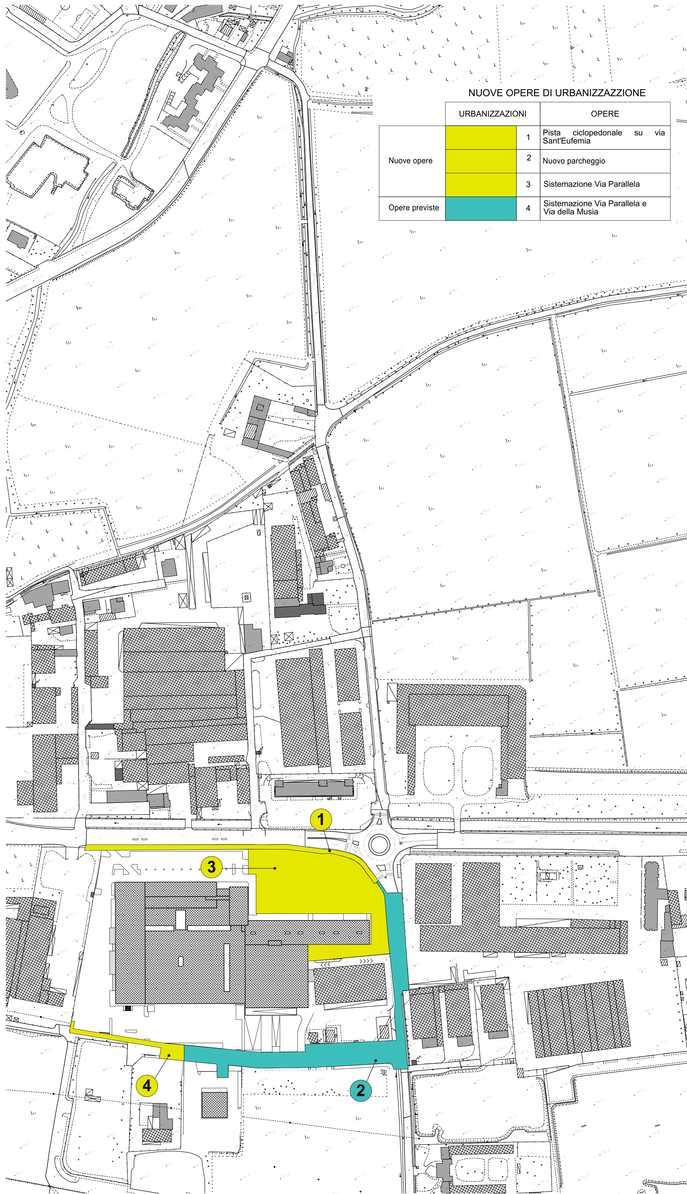
PLANIMETRIA GENERALE OPERE DI URBANIZZAZIONE DA REALIZZARE
