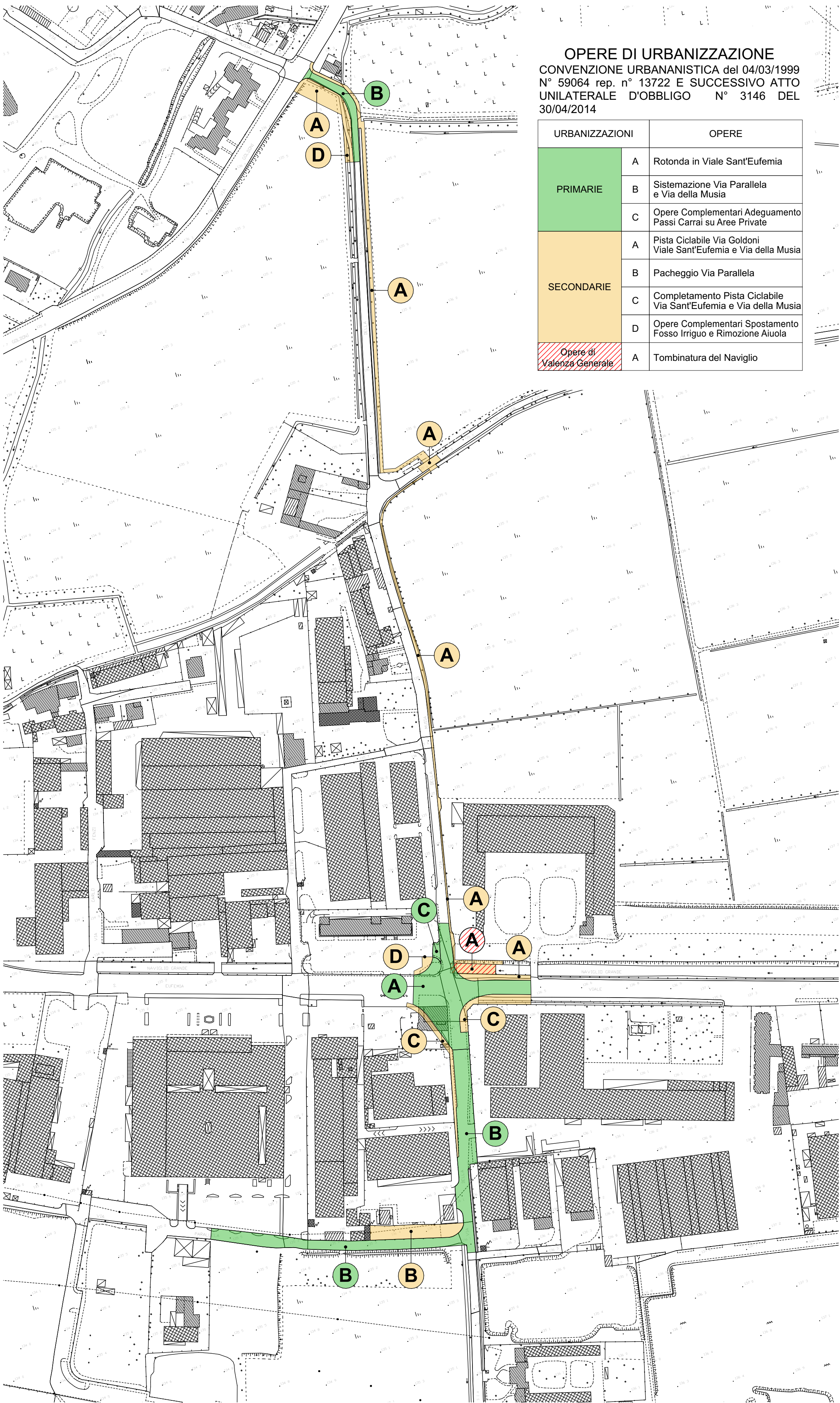
PLANIMETRIA GENERALE OPERE DI URBANIZZAZIONE PREVISTE IN CONVENZIONE
