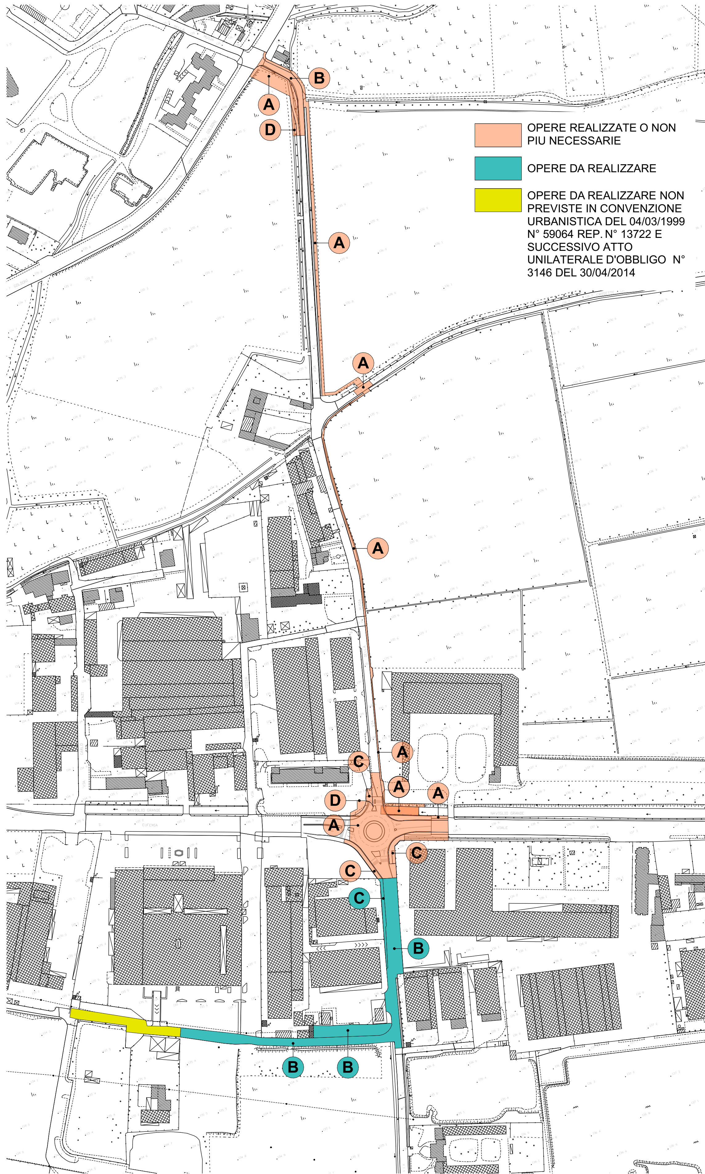
PLANIMETRIA GENERALE DI CONFRONTO OPERE DI URBANIZZAZIONE
